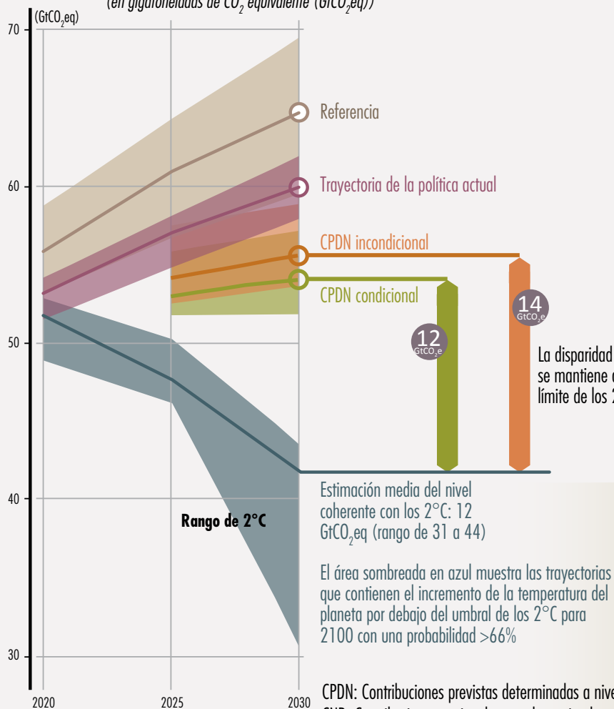
IND T.9.1 Emisiones globales anuales de gases de efecto invernadero (GEI) bajo diferentes escenarios y brechas de emisiones en 2030 (en gigatoneladas de CO 2 equivalente (GtCO 2 eq))
